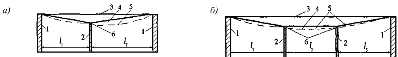
Рисунок 1 – Схеми для визначення значень l ( l_1 , l_2 , l_3 ) за наявності між стінами капітальних перегородок: а) однієї в прогоні; б) двох у прольоті; 1 – несучі стіни (колони); 2 – капітальні перегородки; 3 – перекриття (покриття) до прикладення навантаження; 4 – перекриття (покриття) після прикладення навантаження; 5 – лінії відліку прогинів; 6 – зазор
