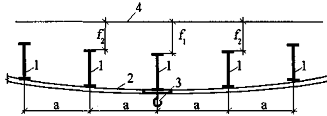
Рисунок 2 – Схема для визначення прогинів кроквяних конструкцій при наявності кранових колій: 1 – кроквяні конструкції; 2 – балка підвісної кранової колії; 3 – підвісний кран; 4 – вихідне положення кроквяних конструкцій; f_1 – прогин найбільш навантаженої кроквяної конструкції; f_2 – прогини кроквяних конструкцій, суміжних з найбільш навантаженою кроквяною конструкцією.
