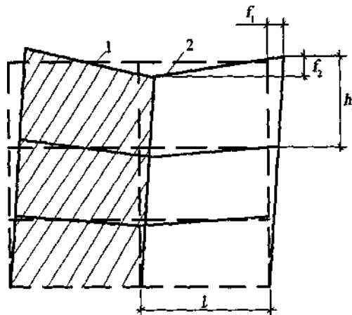
Рисунок 3 – Схема перекошу поверхових комірок (2), що примикають до діафрагм жорсткості (1) у будівлях зі зв'язевим каркасом (пунктиром показана схема каркаса до прикладення навантаження)
