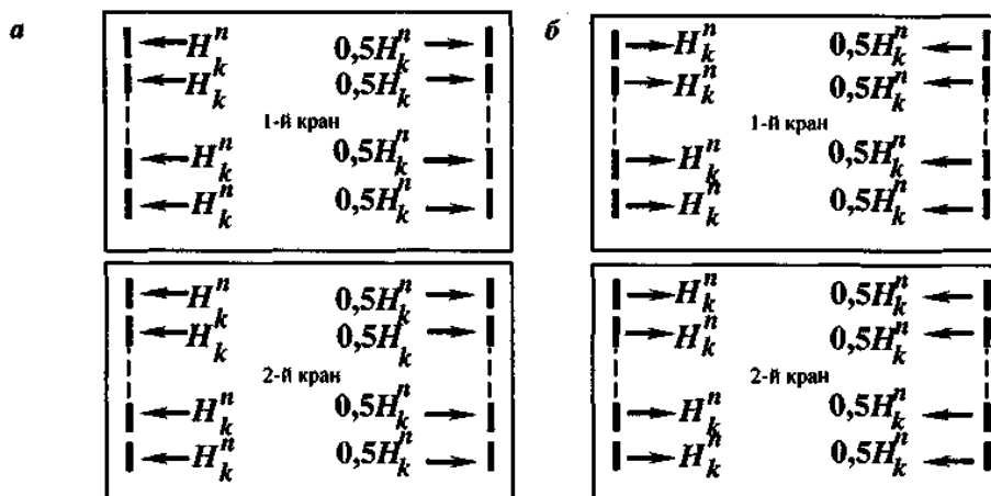
Рисунок 7.2. Варіанти прикладення бічних сил для багатоколісних кранів
