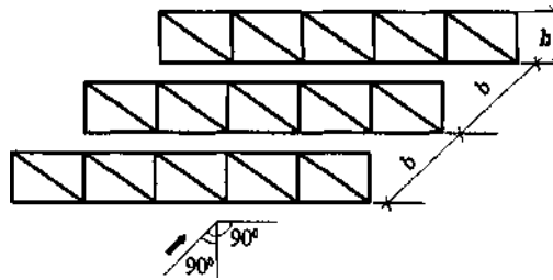
Схема 17. Ряд плоских паралельно розташованих гратчастих конструкцій
