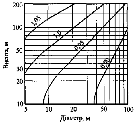
Рисунок 9.7. Коефіцієнт C_d для будівель із сталебетонним каркасом
