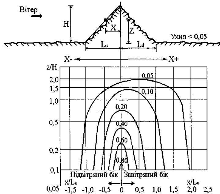
Рисунок 9.4. Коефіцієнт S для пагорбів
