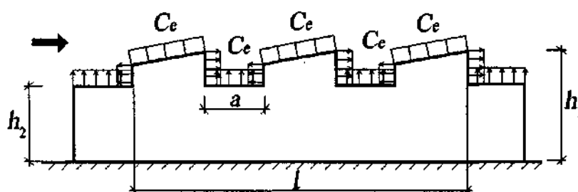
Схема 8. Будівлі з зенітними ліхтарями
