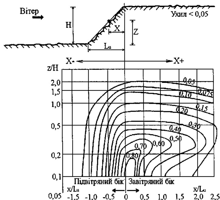
Рисунок 9.3. Коефіцієнт S для схилів
