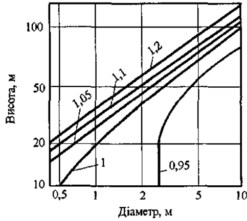
Рисунок 9.10. Коефіцієнт C_d для залізобетонних труб
